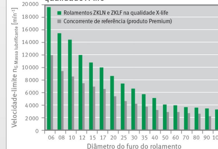
Maiores velocidades-limite graças à qualidade X-life
