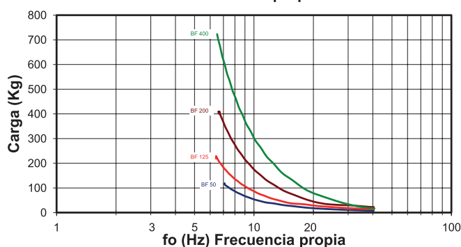
Frecuencia propia
