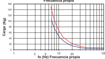
Frecuencia propia
