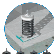
Vibrabsorber + Sylomer®
