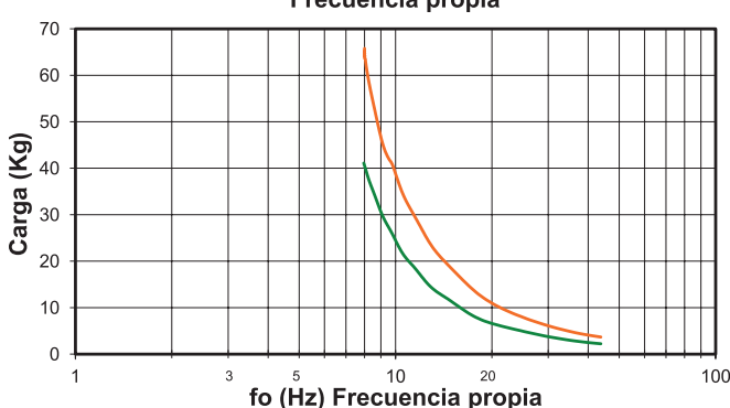
Frecuencia propia
