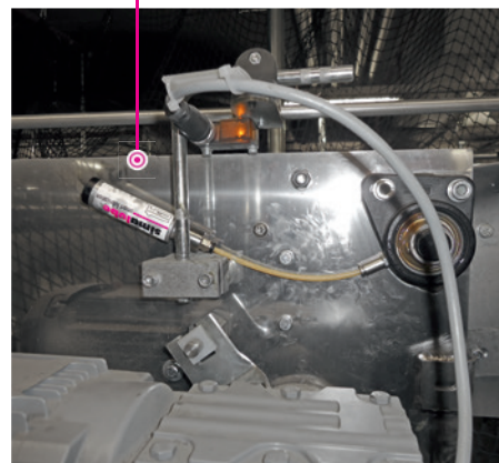
Lubrificação de rolamento com flange com simalube 15 ml, o lubrificador mais pequeno do mundo.
