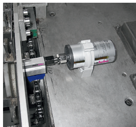
Na indústria alimentar são utilizadas escovas especiais com cerdas azuis, porque podem ser detetadas mais facilmente pelas camaras de monitorização.
